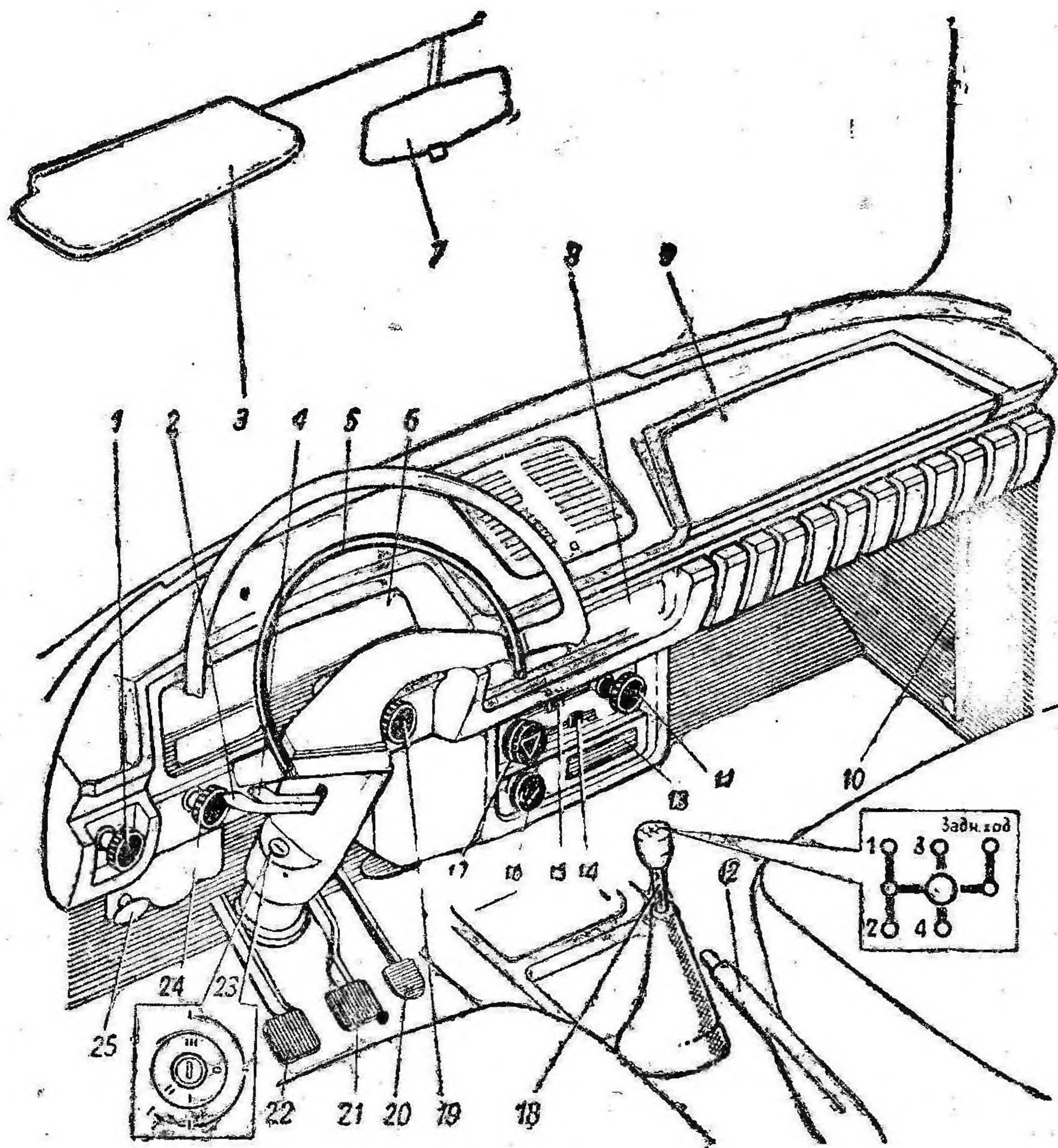
Рис. 5. Органы управления:
