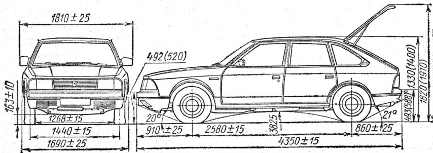
Рис. 1. Автомобиль «АЗЛК-2141»
