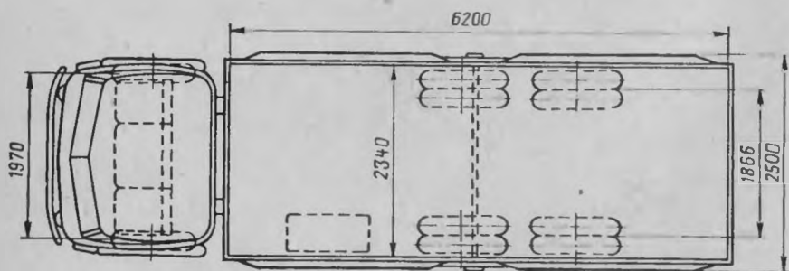
Автомобиль МАЗ-516Б
