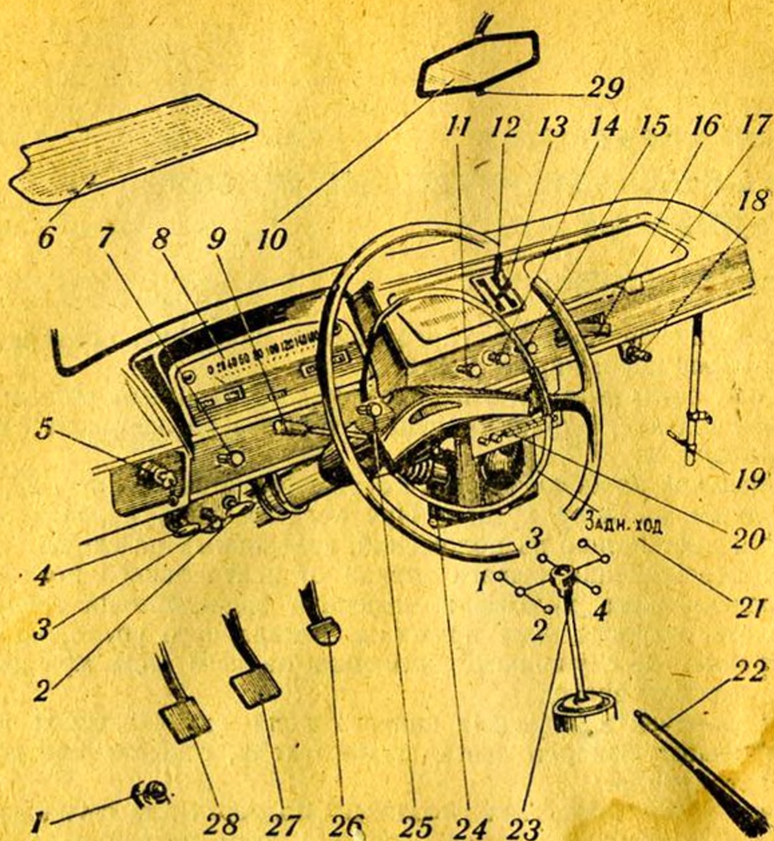
Рис. 3. Органы управления:
