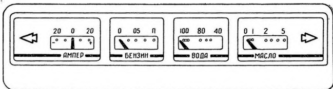
Фиг. 5. Комбинация приборов автомобиля М-72.
