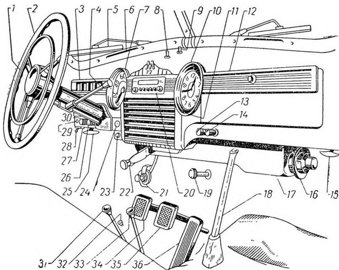
Фиг. 4. Органы управления и приборы автомобиля М-72:
