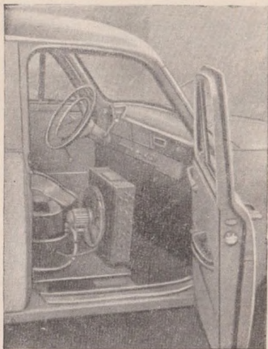
Рис. 10. Расположение холодильных агрегатов в автомобиле-рефрижераторе
