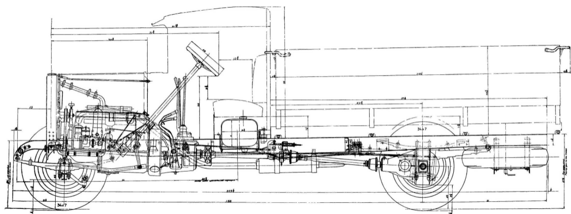
Чертеж 45.
