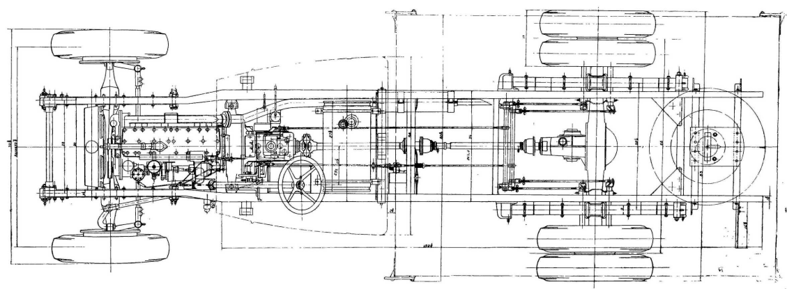
Чертеж 46.
