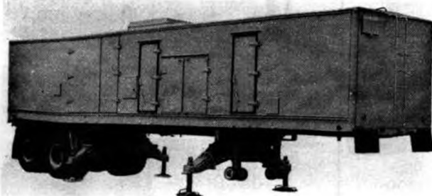
ОдАЗ-9987. Фургон для газотурбинной электростанции мощностью 2500 кВт
