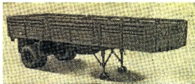
Полуприцеп МАЗ-5245
