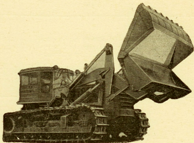
Рис. 2. Универсальный одноковшовый погрузчик Д-543 в работе
