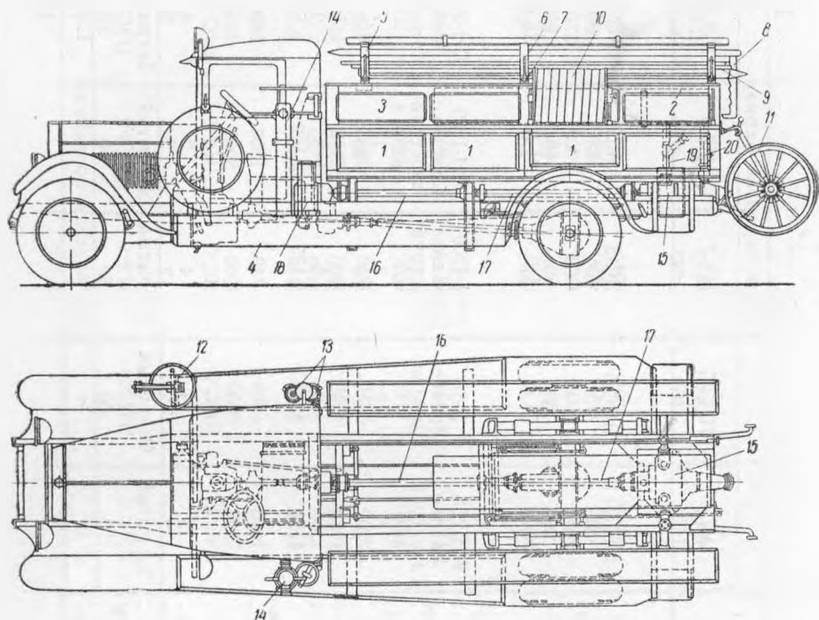
Рис. 121. Автонасос ПМЗ-1:
