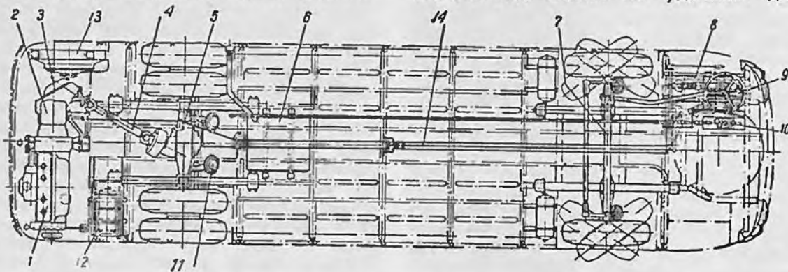
Рис. 1. Общая компоновка автобуса ЗИС-127
