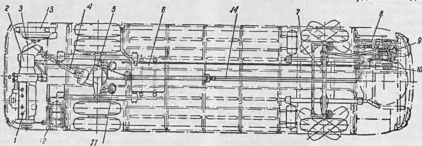
Рис. 1. Общая компоновка автобуса ЗИС-127
