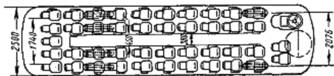
Схема автобуса ЛАЗ-699А
