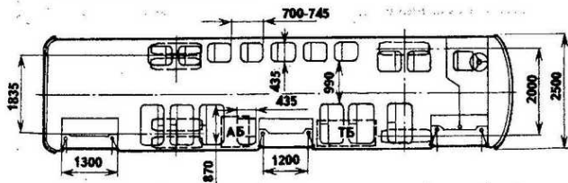
Автобус IKARUS-260.50 4×2.2
